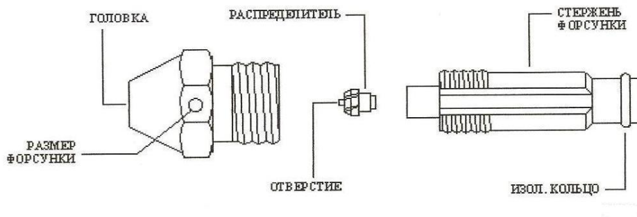
Рис. 25. Устройство форсунки .
