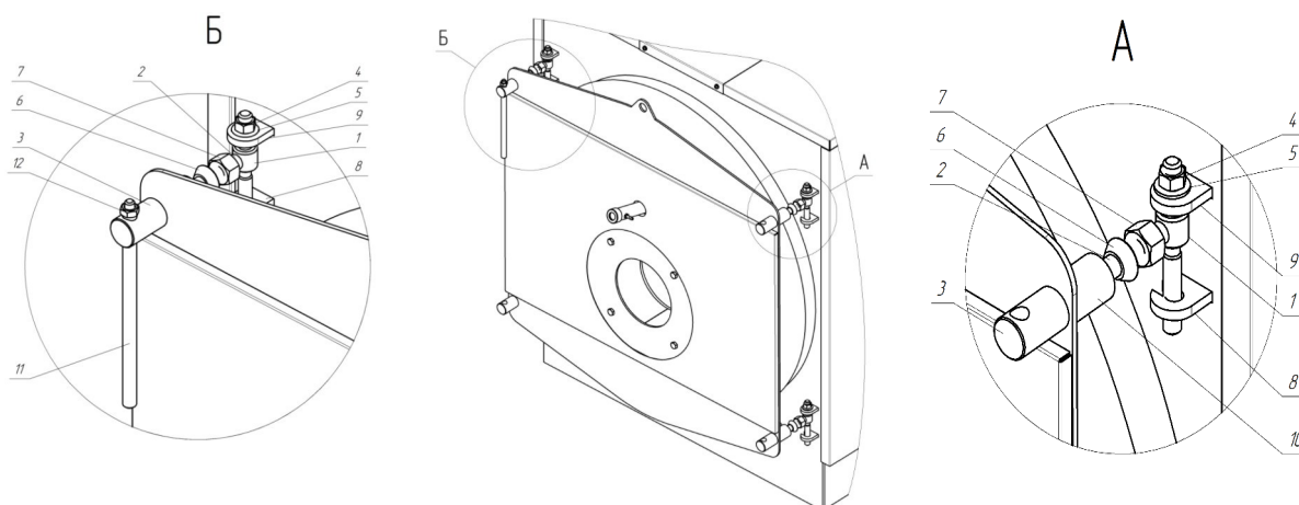
Рисунок 9. Петли передней дверцы
