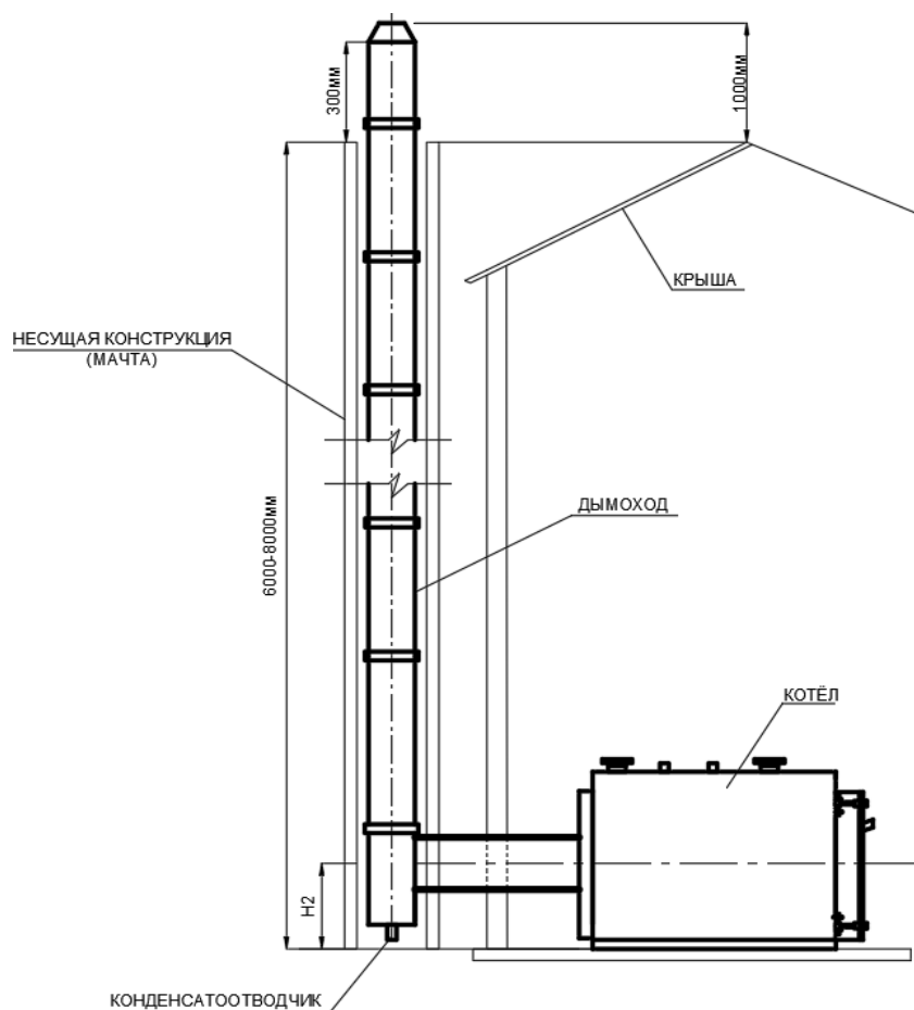
Рисунок 8.1 Вариант дымохода на несущей конструкции
