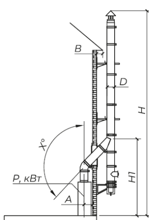
Рисунок 8.2 Варианты дымоходов по зданию
