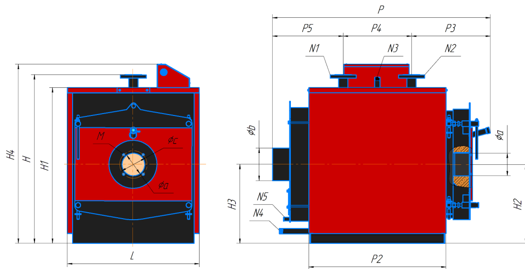
Рисунок 2. Габаритные размеры котлов моделей от V 500 до V 3000
