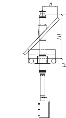
Рисунок 8.2 Варианты дымоходов по зданию
