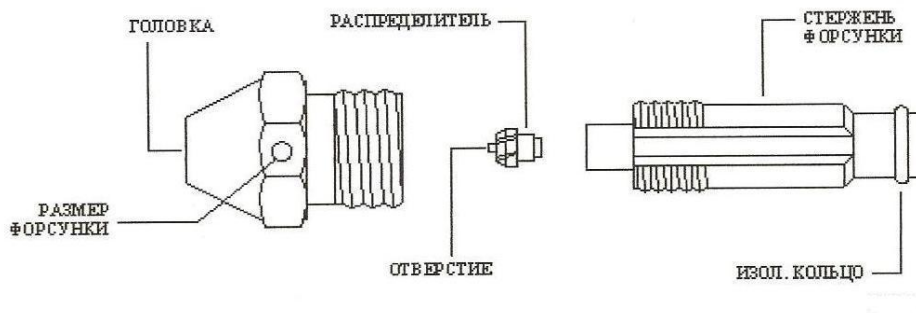
Рис. 25. Устройство форсунки.
