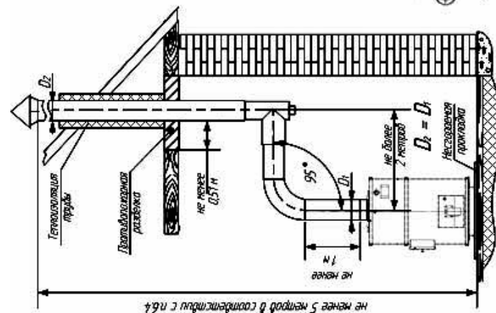
Схема № 2 установка дымовой трубы с выводом через потолочное перекрытие
