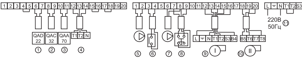
Рис. 7.2: Электрическая схема подключения внешних устройств
