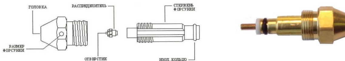
Рис. 23 Устройство форсунки.
