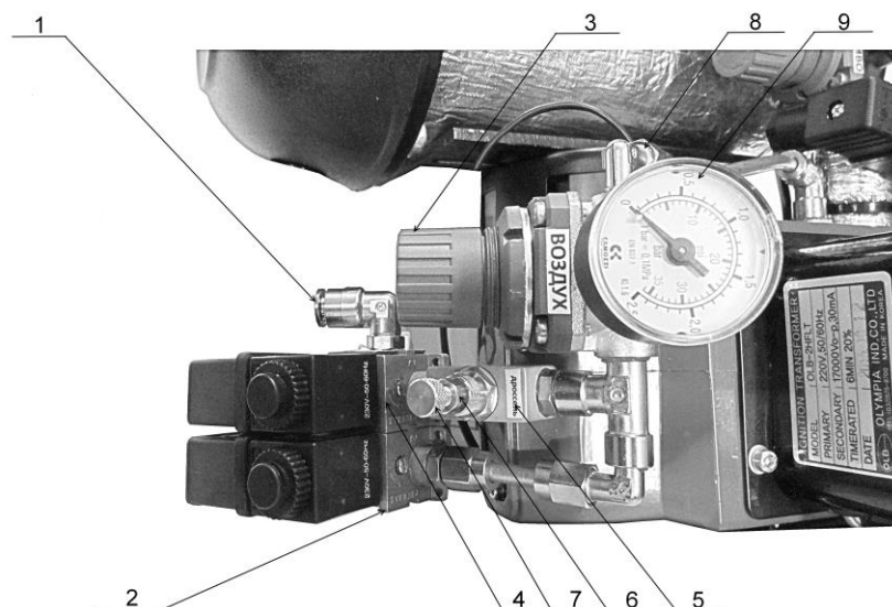
Рис. 11. Подача первичного воздуха.
